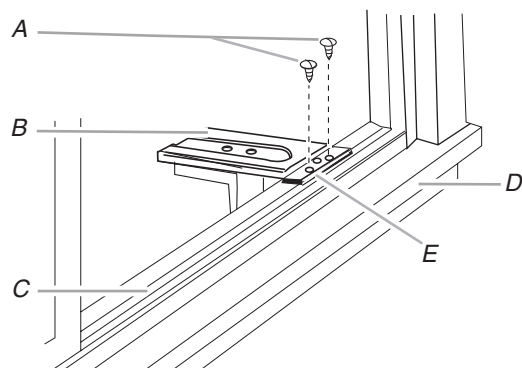
A. Tornillos para madera de 1" B. Placa de soporte C. Riel inferior de la ventana D. Repisa de la ventana E. Tira espaciadora
