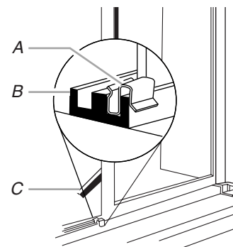
A. Pincas rapides B. Rainure de fenêtre C. Joint en plastique
