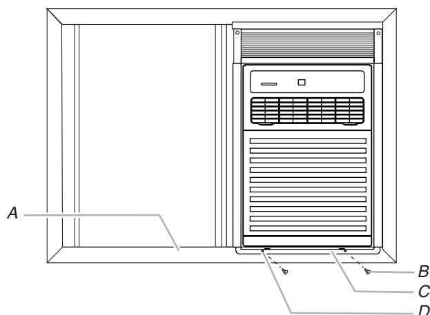
A. Marco del canal de la ventana B. Tornillo autorroscante de \frac{3}{8} " C. Soporte inferior D. Orificio taladrado de \frac{1}{8} "
